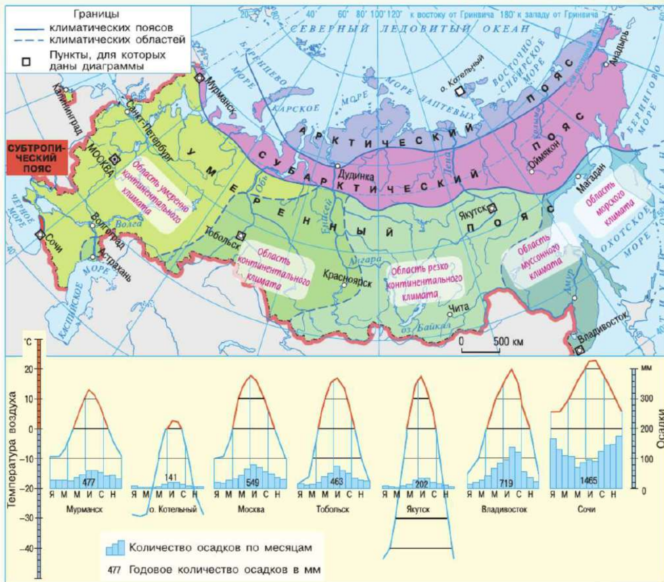
Рис. 55. Климатические поясы и области России
