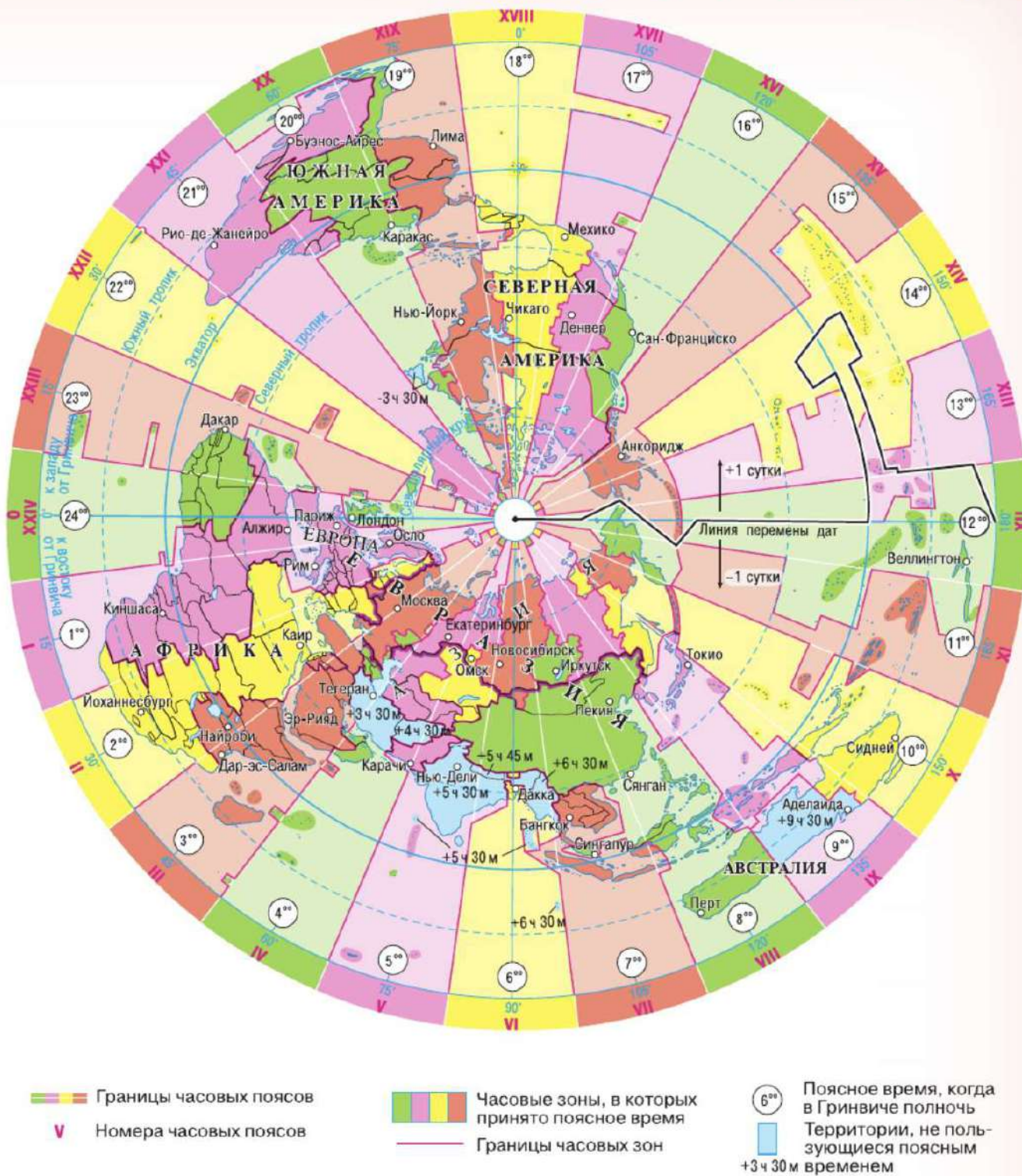
Рис. 3. Часовые пояса и зоны мира
