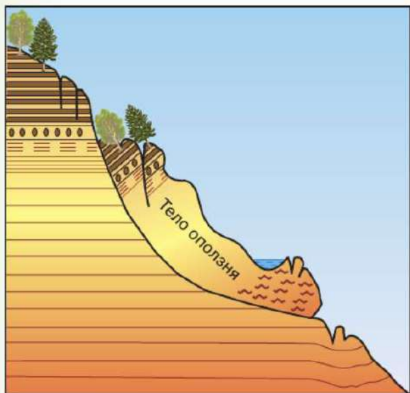
Рис. 40. Образование оползня
