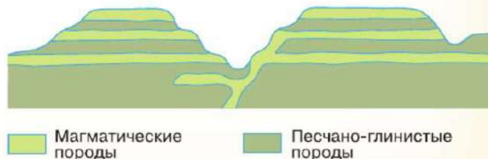
Рис. 83. Траппы Восточной Сибири
