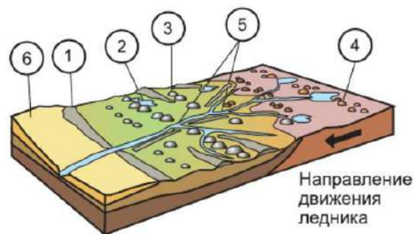
Рис. 32. Ледниковые формы рельефа: 1 — конечная моренная гряда; 2 — озеро, подпруженное мореной; 3 — моренный холм; 4 — бараньи лбы (оглаженные ледником выступы скальных пород); 5 — озы; 6 — зандровая равнина
