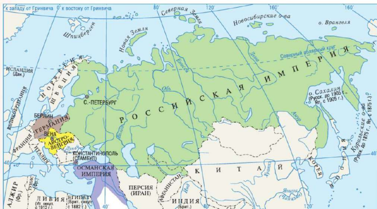
Рис. 7. Российская, Османская, Австро-Венгерская и Германская империи в начале XX в.
