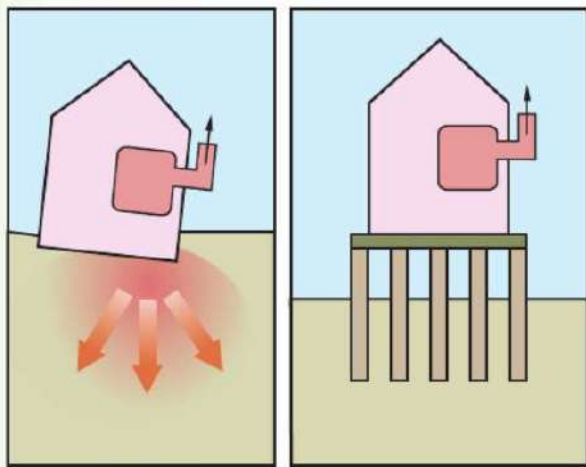
Рис. 41. Как возводить постройки на многолетней мерзлоте
