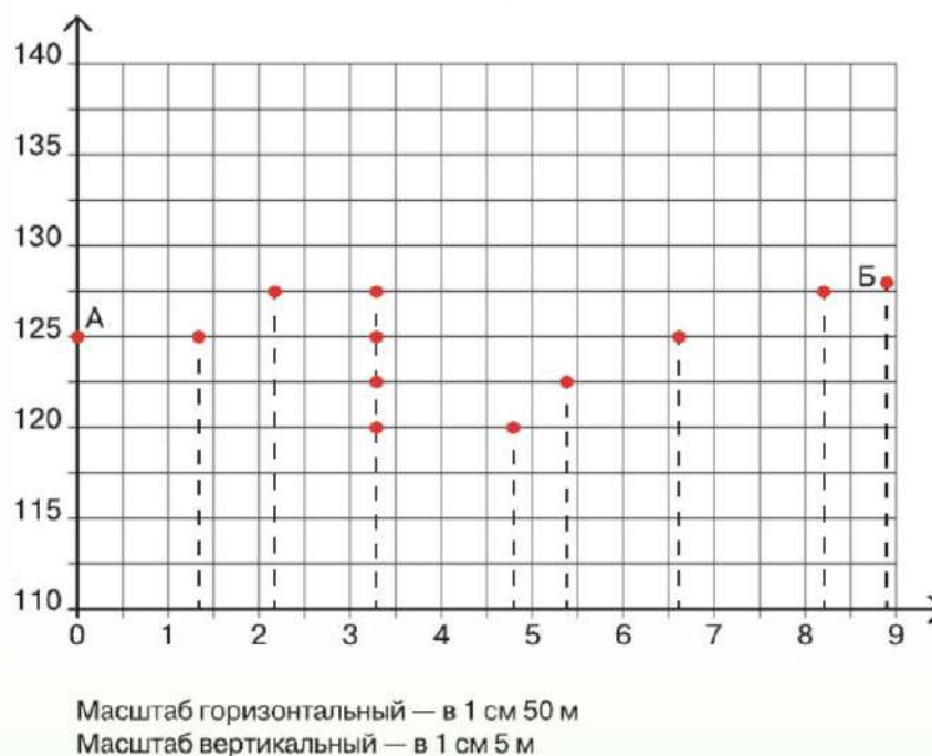
Рис. 37. Перенос высот на основу
