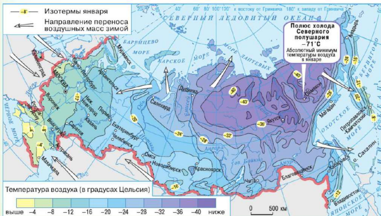
Рис. 50. Средние температуры воздуха в январе
