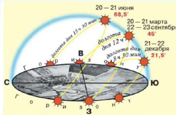
Рис. 44. Высота Солнца над горизонтом и продолжительность дня на параллели 45^\circ с. ш.
