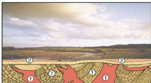
Рис. 29. Строение платформы: 1 — кристаллический фундамент; 2 — осадочный чехол
