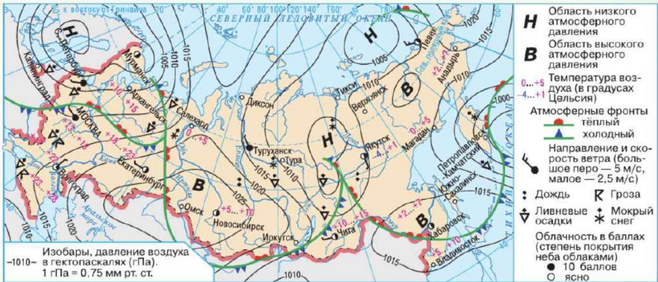
Рис. 54. Синоптическая карта
