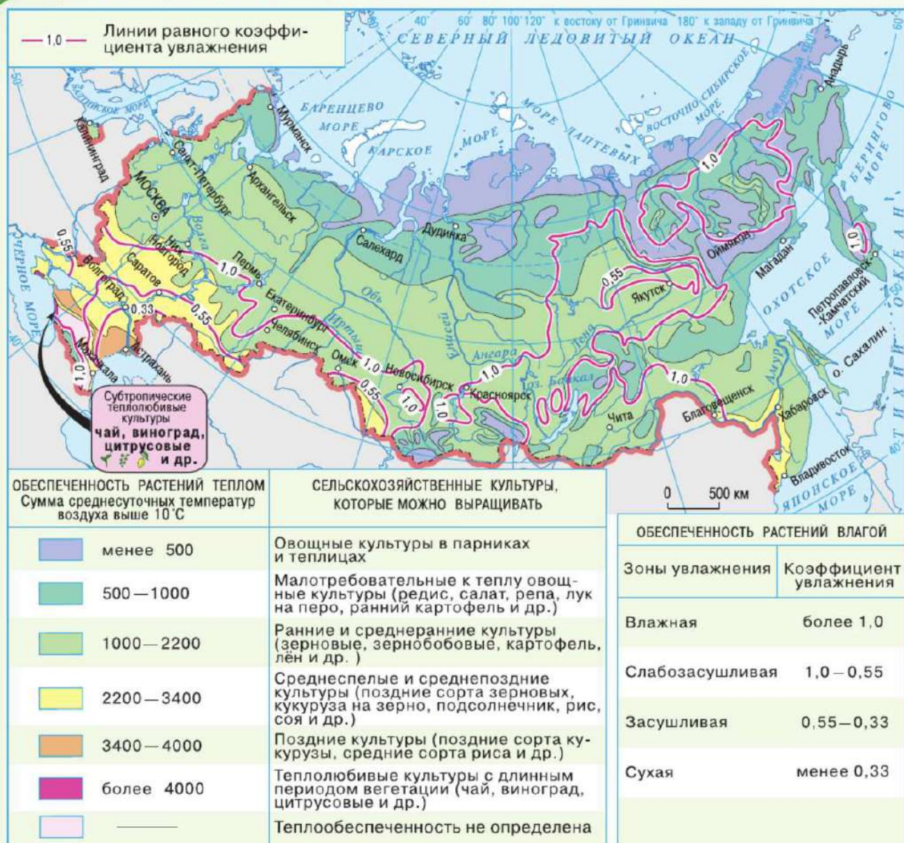
Рис. 58. Агроклиматические ресурсы
