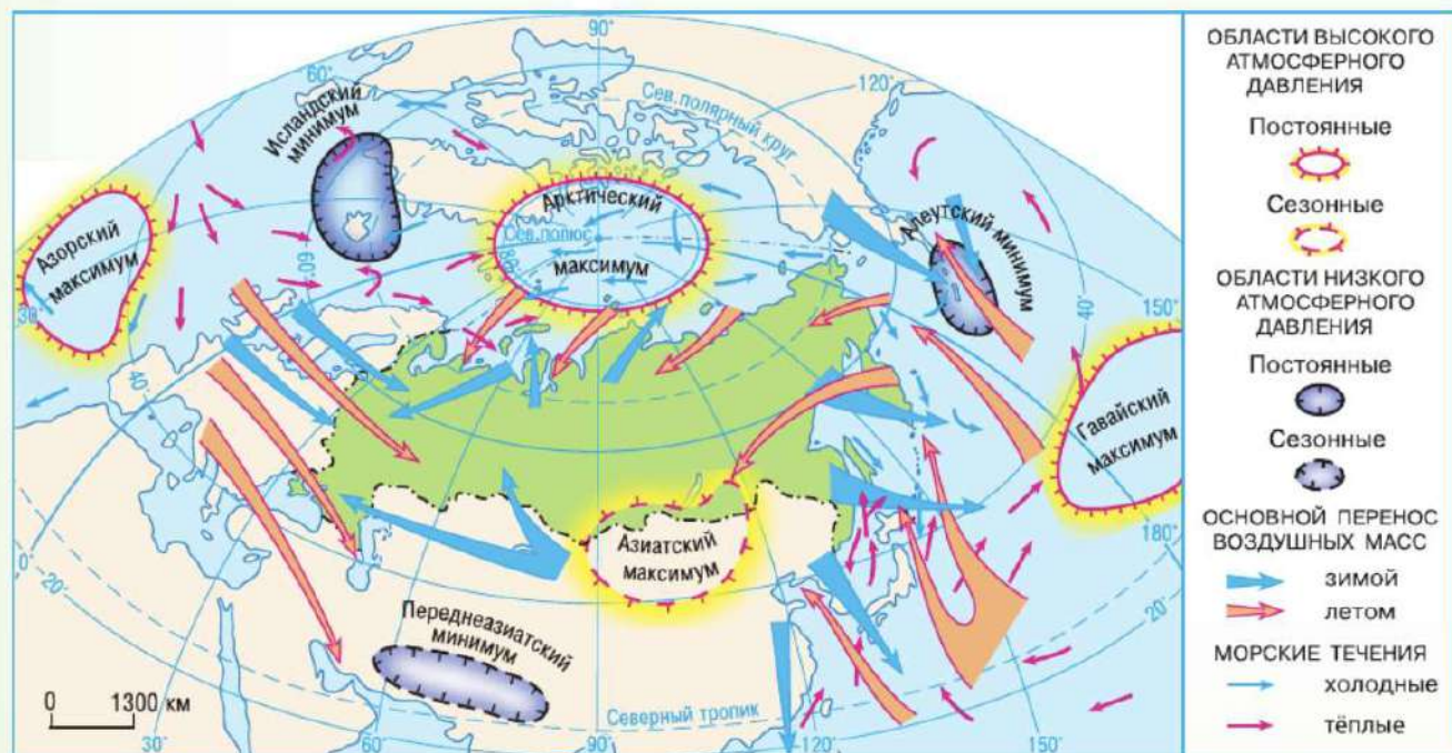
Рис. 45. Влияние соседних территорий на климат России
