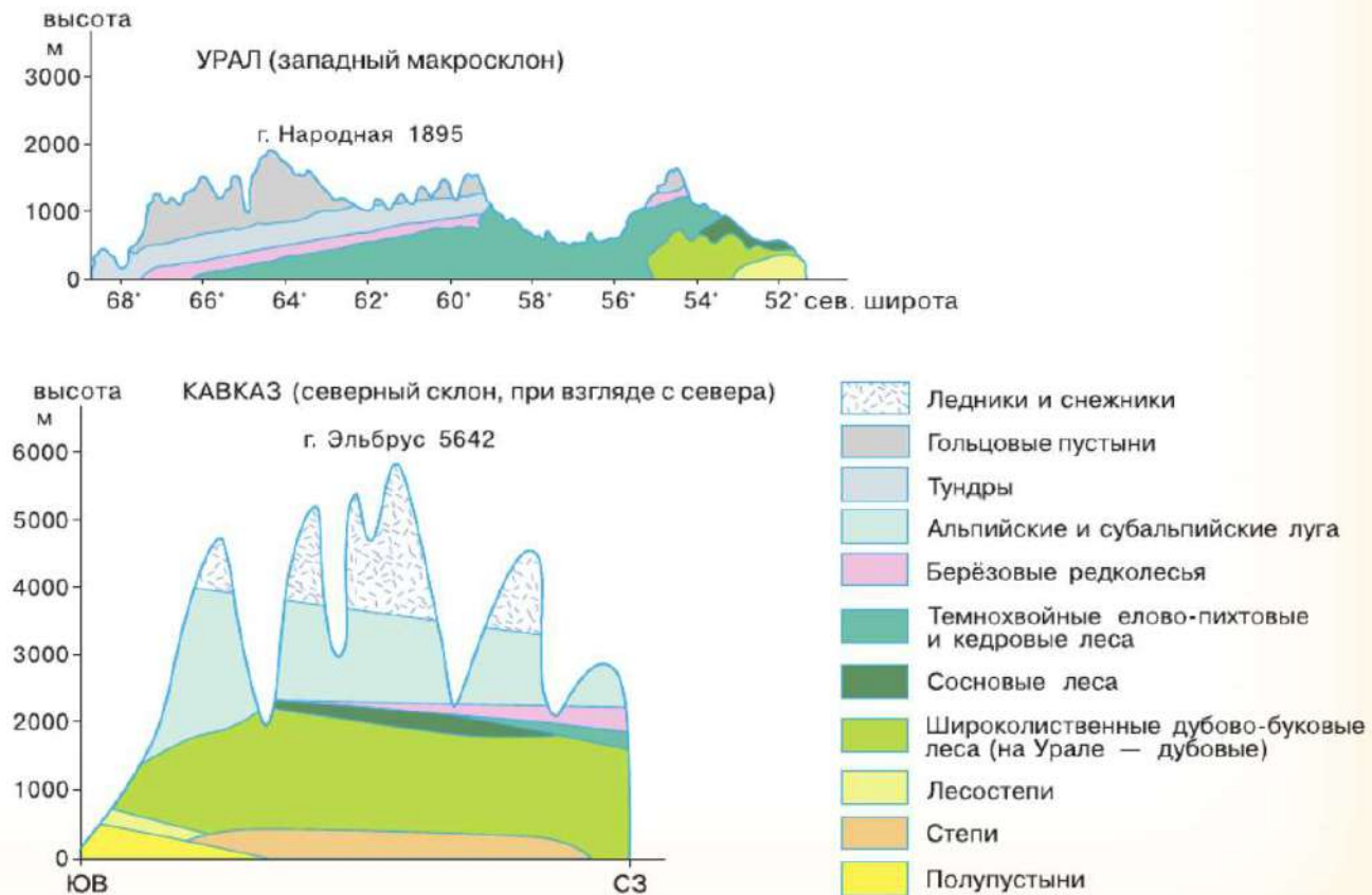
Рис. 79. Высотная поясность
