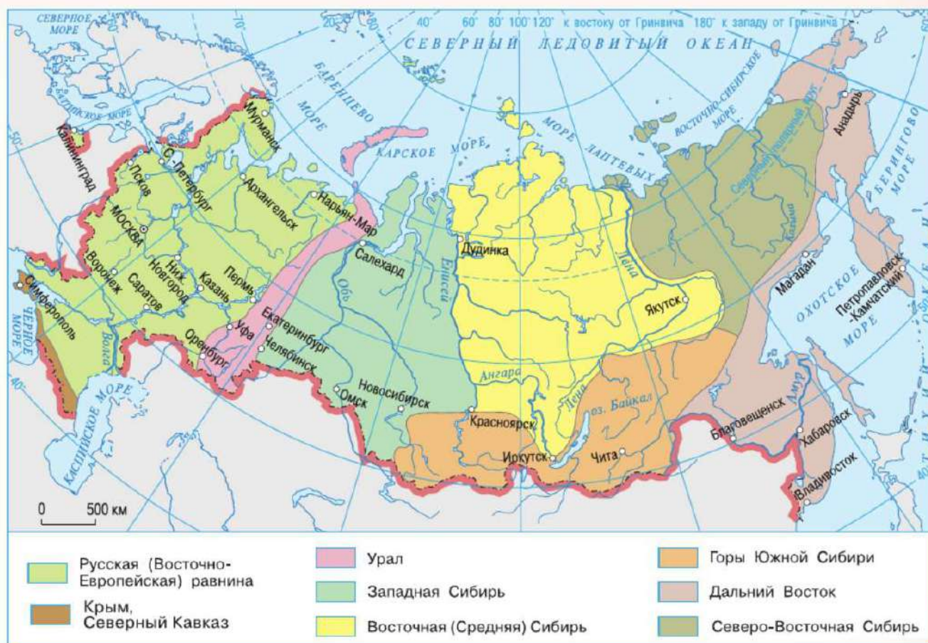
Рис. 10. Природные районы России
