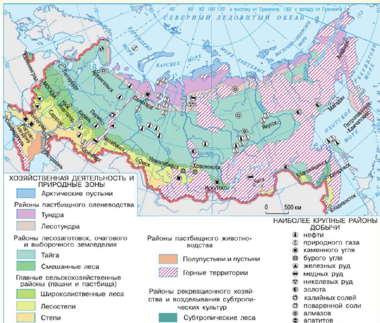
Рис. 80. Природно-хозяйственные зоны России
