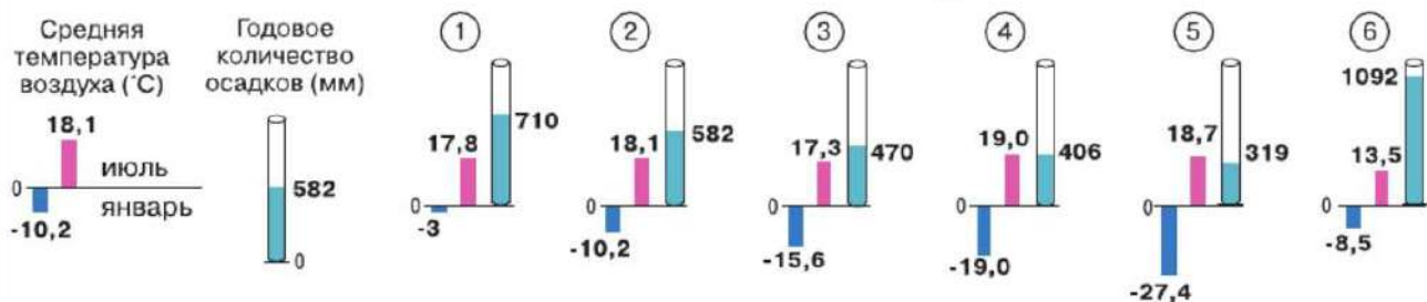
ИЗМЕНЕНИЕ КЛИМАТИЧЕСКИХ ПОКАЗАТЕЛЕЙ С ЗАПАДА НА ВОСТОК
