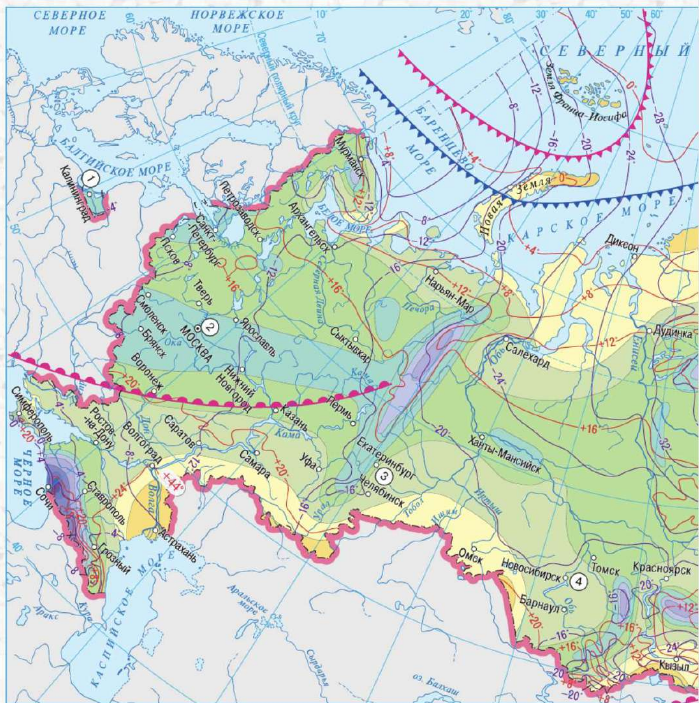
ИЗМЕНЕНИЕ КЛИМАТИЧЕСКИХ ПОКАЗАТЕЛЕЙ С ЗАПАДА НА ВОСТОК
